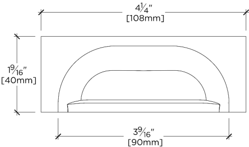
FRONT VIEW SCALE: 6"=1'-0"
