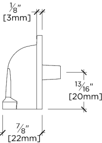
SIDE VIEW SCALE: 6"=1'-0"
