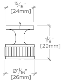
TOP VIEW SCALE: 6"=1'-0"
