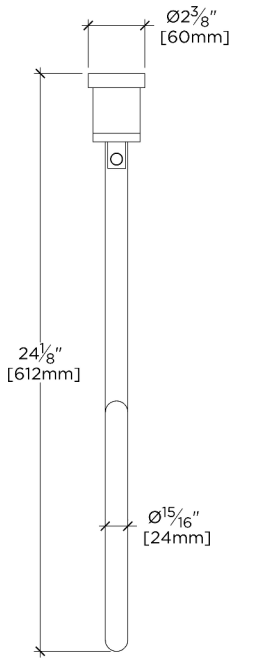
TOP VIEW SCALE: 1\frac{1}{2}"=1'-0"
