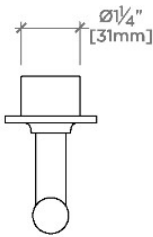
TOP VIEW SCALE: 3"=1'-0"
