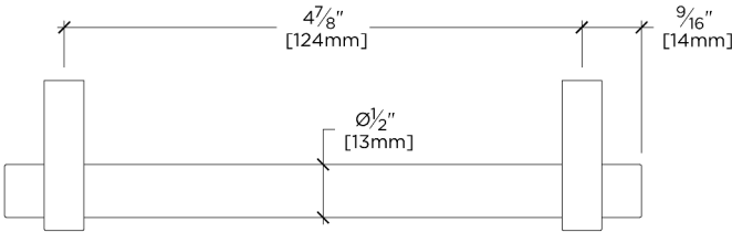
TOP VIEW SCALE: 6"=1'-0"
