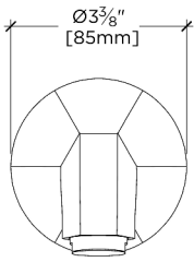
FRONT VIEW SCALE: 3"=1'-0"
