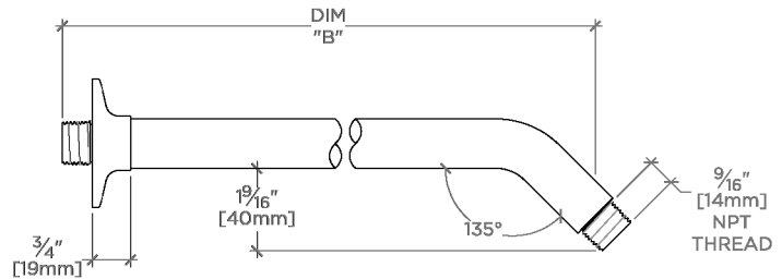
SIDE VIEW SCALE: 3"=1'-0"
