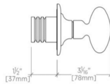
SIDE VIEW SCALE: 3"=1'-0"
