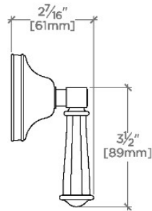
SIDE VIEW SCALE: 3"=1'-0"
