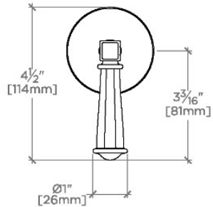
FRONT VIEW SCALE: 3"=1'-0"
