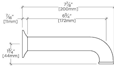
SIDE VIEW SCALE: 3"=1'-0"
