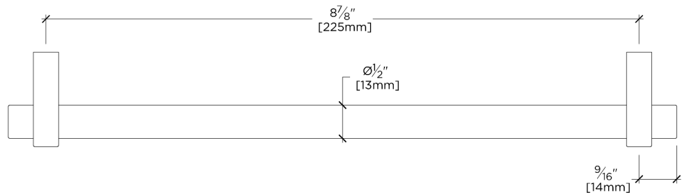
TOP VIEW SCALE: 6"=1'-0"
