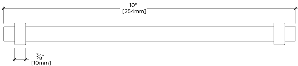
FRONT VIEW SCALE: 6"=1'-0"
