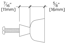
SIDE VIEW SCALE: 6"=1'-0"
