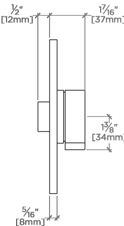
SIDE VIEW SCALE: 3"=1'-0"
