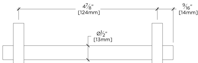
TOP VIEW SCALE: 6"=1'-0"
