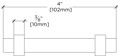
FRONT VIEW SCALE: 6"=1'-0"
