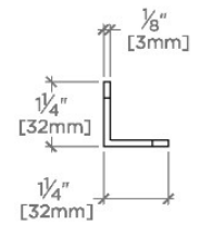
SIDE VIEW SCALE: 3"=1'-0"
