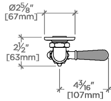
TOP VIEW SCALE: 1\frac{1}{2}"=1'-0"
