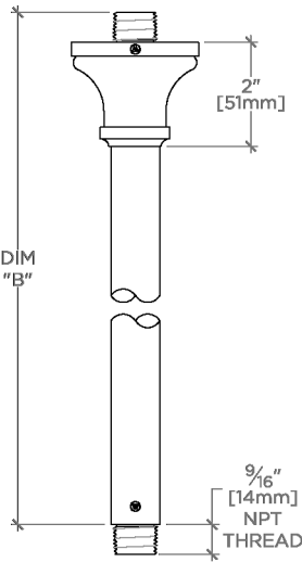
SIDE VIEW SCALE: 3"=1'-0"
