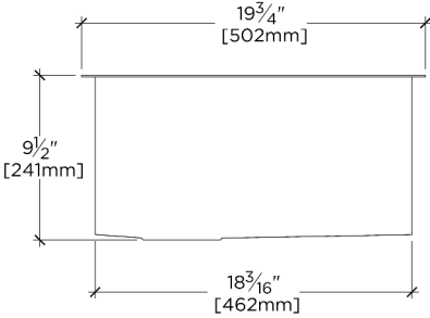
SIDE VIEW SCALE: 1"=1'-0"
