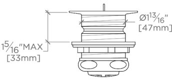
SIDE VIEW SCALE: 3"=1'-0"
