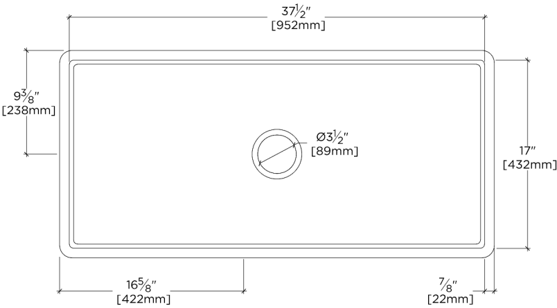
TOP VIEW SCALE: 1"=1'-0"
