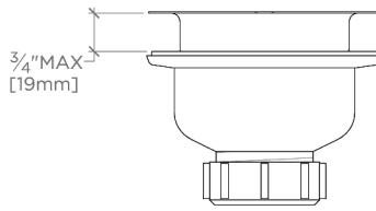
SIDE VIEW SCALE: 3"=1'-0"
