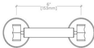
FRONT VIEW SCALE: 3"=1'-0"
