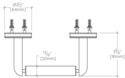
TOP VIEW SCALE: 3"=1'-0"
