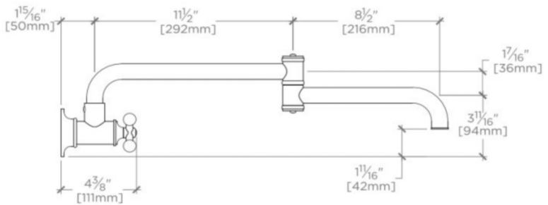
SIDE VIEW SCALE: 1½"=1'-0"
