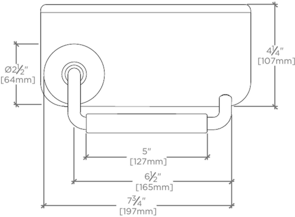
FRONT VIEW SCALE: 3"=1'-0"
