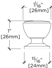
FRONT VIEW SCALE: 6"=1'-0"
