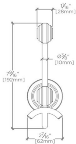
FRONT VIEW SCALE: 3"=1'-0"
