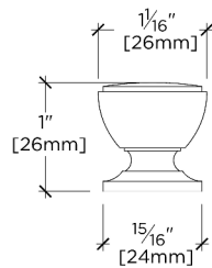
FRONT VIEW SCALE: 6"=1'-0"
