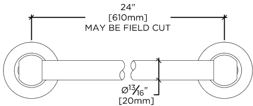
FRONT VIEW SCALE: 3"=1'-0"
