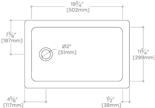
TOP VIEW SCALE: 1"=1'-0"
