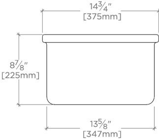
SIDE VIEW SCALE: 1"=1'-0"
