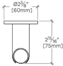
SCALE: 3"=1'-0"
