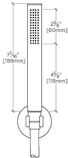
SCALE: 3"=1'-0"
