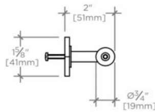
SIDE VIEW SCALE: 3"=1'-0"
