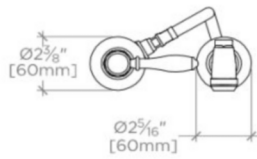
TOP VIEW SCALE: 1\frac{1}{2}"=1'-0"
