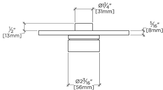
TOP VIEW SCALE: 3"=1'-0"
