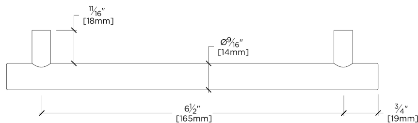
TOP VIEW SCALE: 6"=1'-0"
