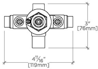
FRONT VIEW SCALE: 3"=1'-0"
