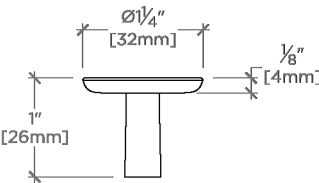
FRONT VIEW SCALE: 6"=1'-0"
