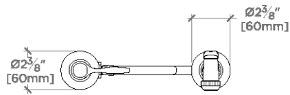
SCALE: 1 1/2"=1'-0"
