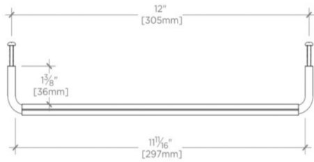
TOP VIEW SCALE: 3"=1'-0"
