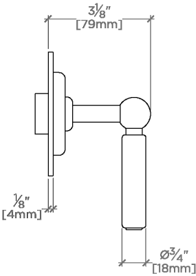
SIDE VIEW SCALE: 3"=1'-0"
