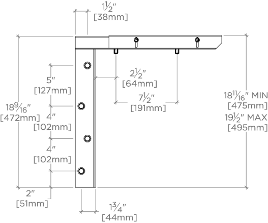
SIDE VIEW SCALE: 1"=1'-0"
