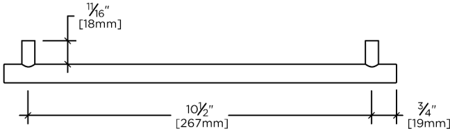
TOP VIEW SCALE: 3"=1'-0"
