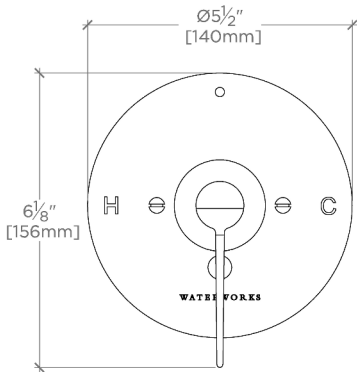
FRONT VIEW SCALE: 3"=1'-0"
