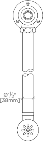
TOP VIEW SCALE: 1 1/2"=1'-0"
