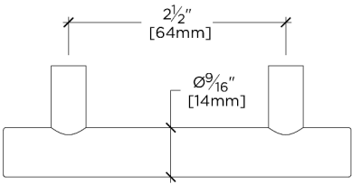
TOP VIEW SCALE: 6"=1'-0"
