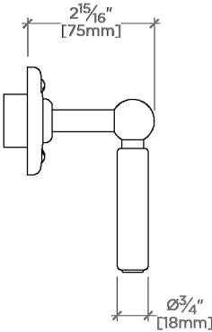
SIDE VIEW SCALE: 3"=1'-0"
