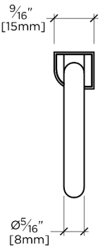
SIDE VIEW SCALE: 6"=1'-0"
