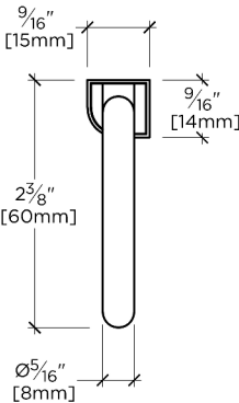
SIDE VIEW SCALE: 6"=1'-0"
