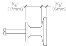
SIDE VIEW SCALE: 6"=1'-0"
