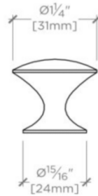
SIDE VIEW SCALE: 6"=1'-0"
